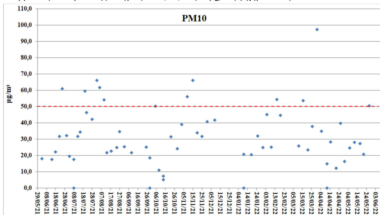
Σχήμα 2.2.1. Ημερήσιες σταθμικές συγκεντρώσεις PM 10 κατά το χρονικό διάστημα 01/06/21-31/05/22
