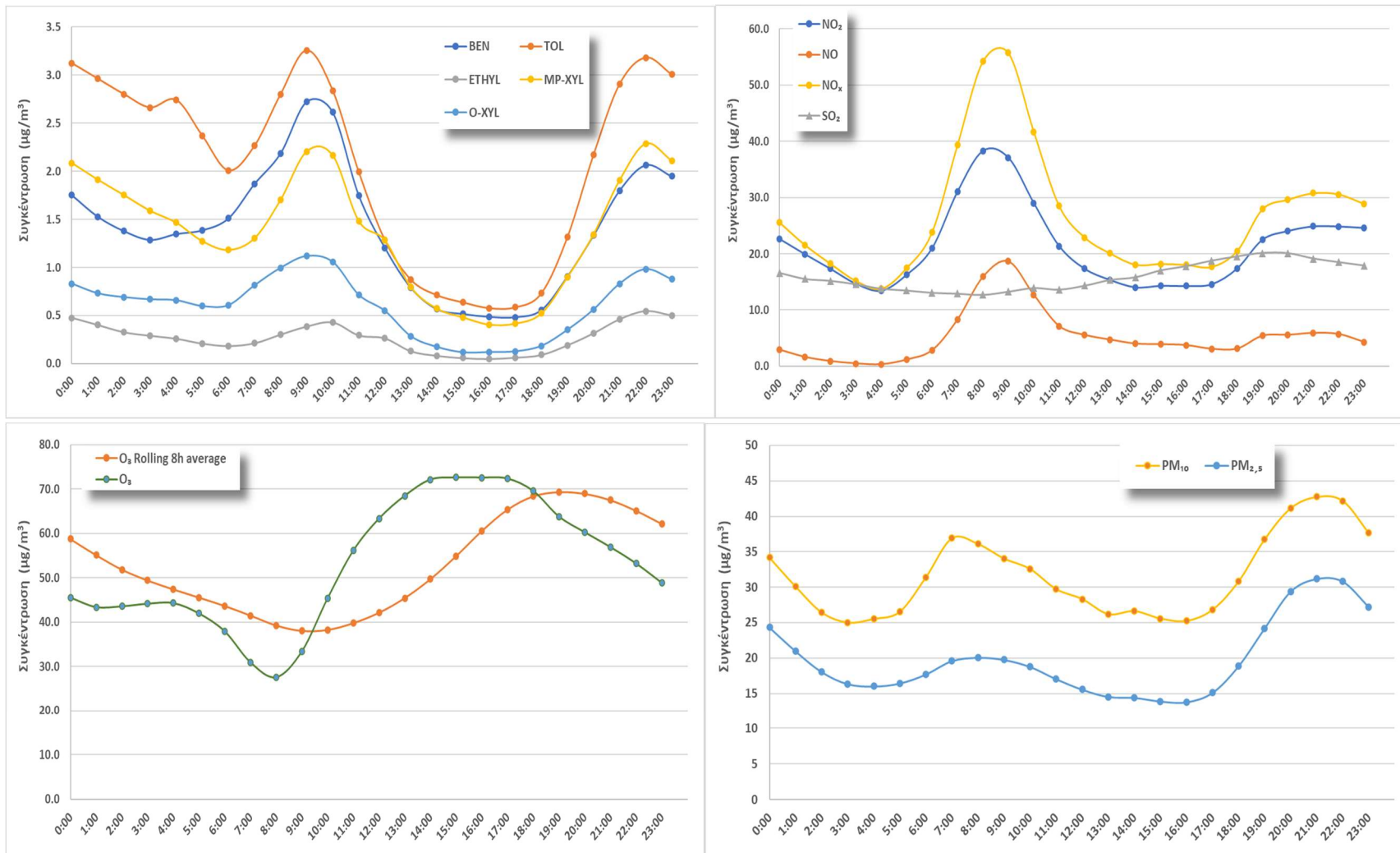
Σχήμα 2.1.1. Μέση ημερήσια διακύμανση των συγκεντρώσεων BTEX, \text{NO}_x , \text{SO}_2 , \text{O}_3 , \text{PM}_{10} και \text{PM}_{2.5} κατά το χρονικό διάστημα 01.06.21-31.05.22
