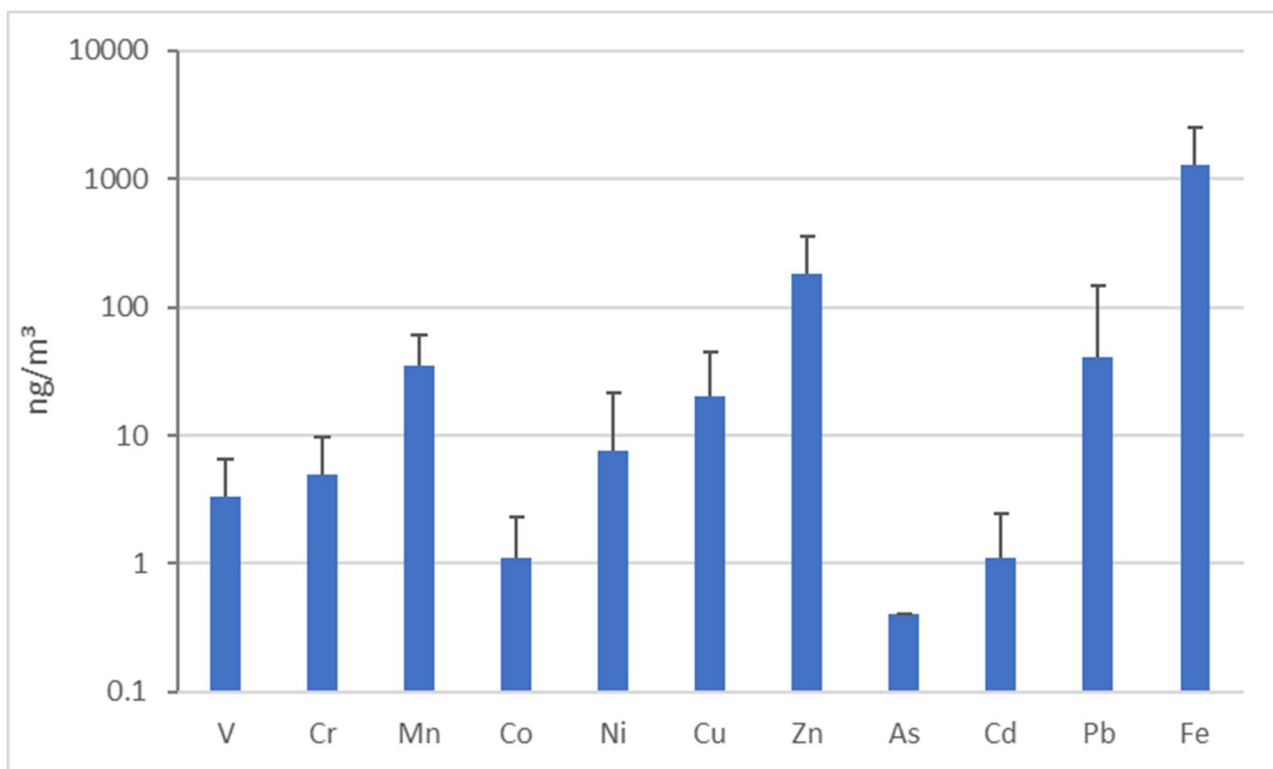
Σχήμα 2.2.3. Μέσες ετήσιες συγκεντρώσεις μετάλλων/μεταλλοειδών κατά το χρονικό διάστημα 01.06.21-31.05.22
