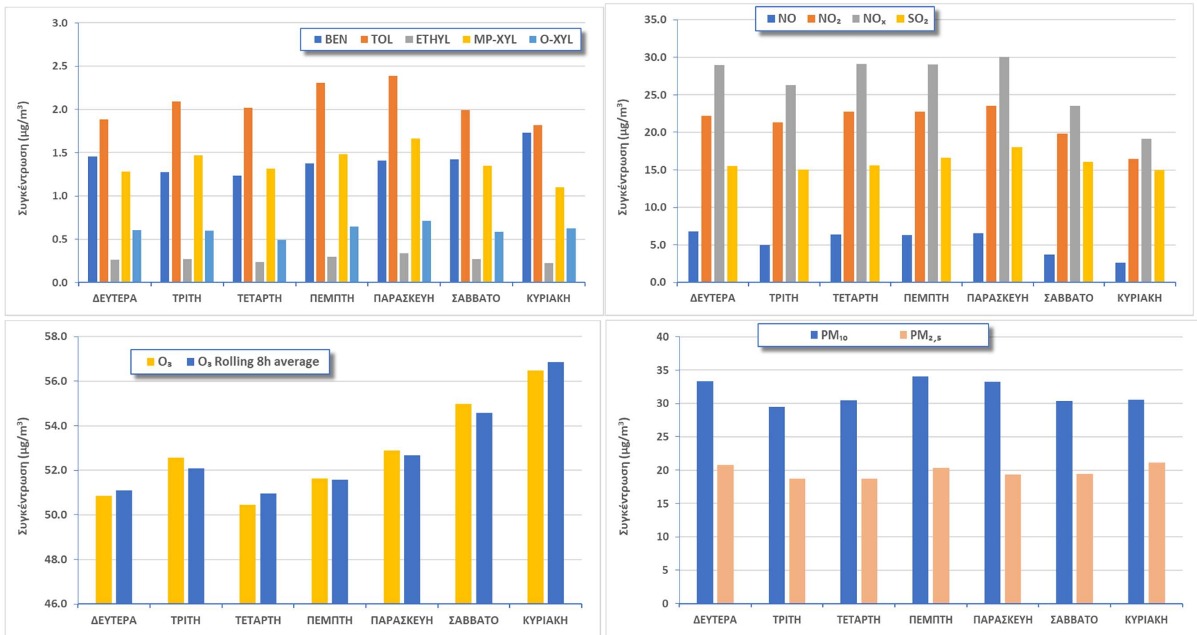
Σχήμα 2.1.2. Μέση εβδομαδιαία διακύμανση των συγκεντρώσεων BTEX, NOx, SO 2 , O 3 , PM 10 και PM 2.5 κατά το χρονικό διάστημα 01.06.21-31.05.22
