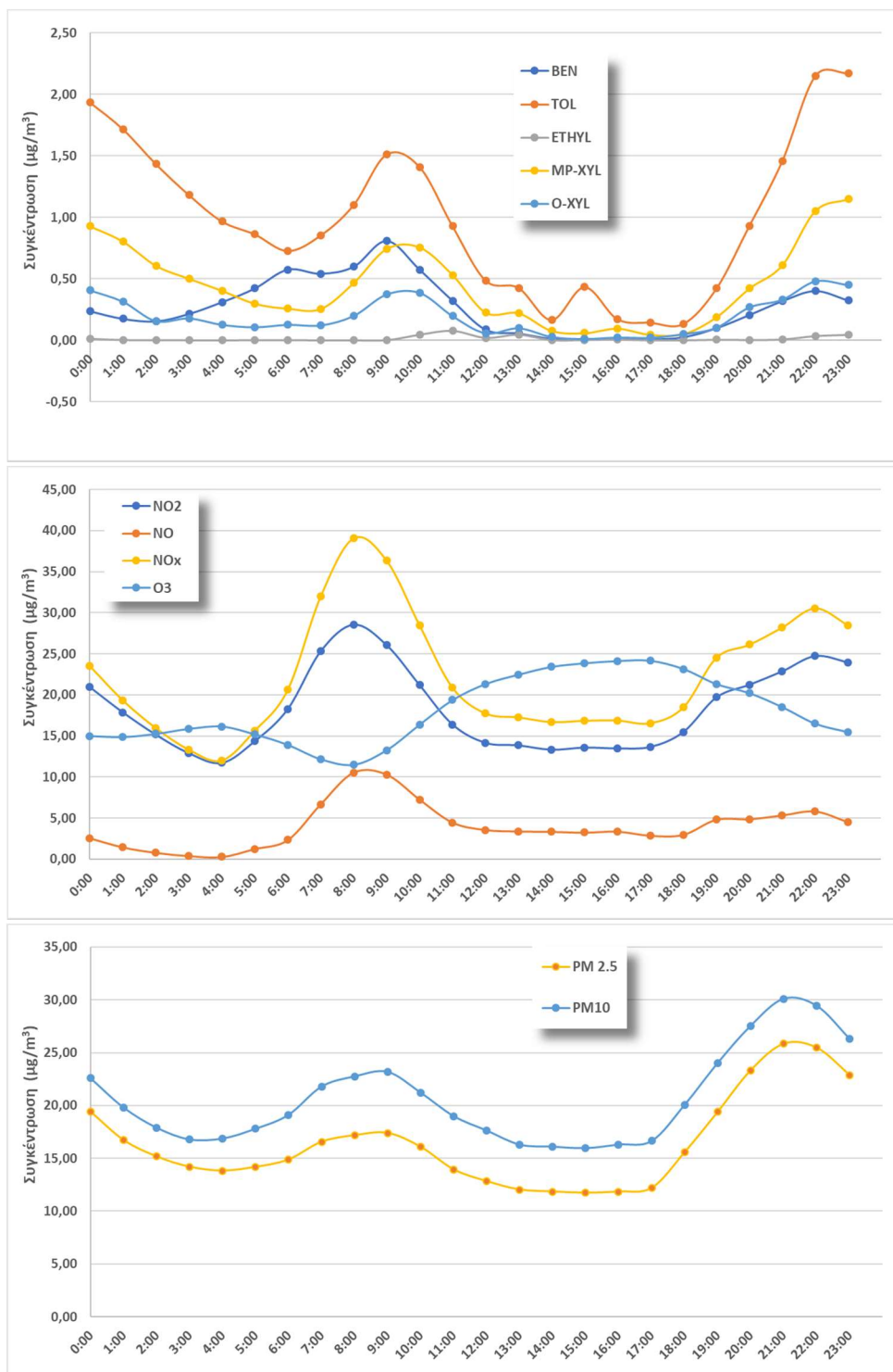
Σχήμα 2.1.1. Μέση ημερήσια διακύμανση των συγκεντρώσεων BTEX, NO x , O 3 , PM 10 και PM 2.5 κατά το χρονικό διάστημα 02/06/2018 – 01/06/2019
