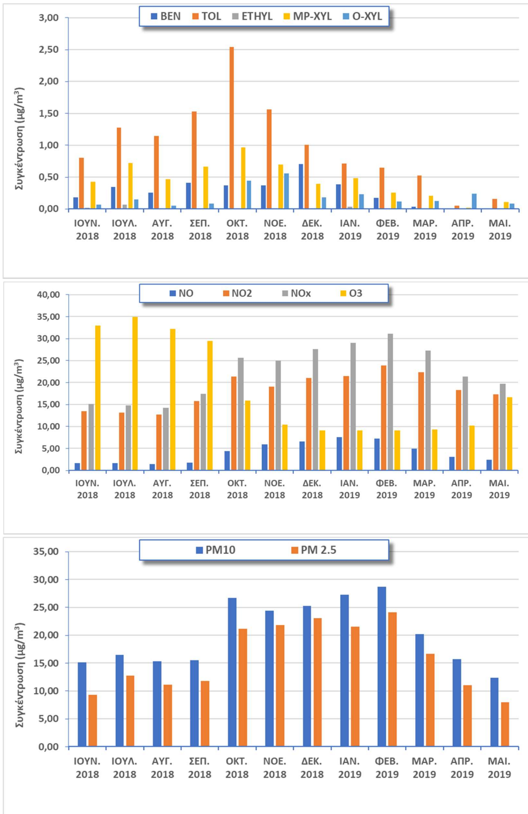
Σχήμα 2.1.3. Μέση μηνιαία διακύμανση των συγκεντρώσεων BTEX, NOx, O 3 , PM 10 και PM 2.5 κατά το χρονικό διάστημα 02/06/2018 – 01/06/2019
