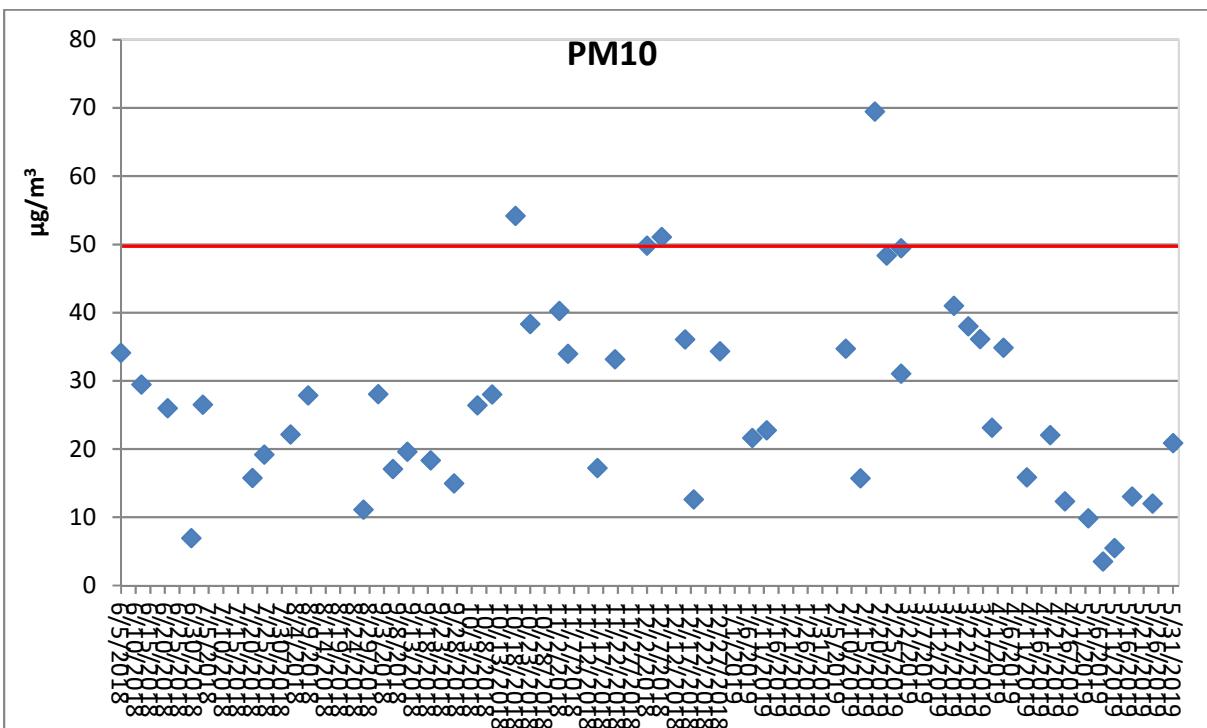
Σχήμα 2.2.1. Ημερήσιες σταθμικές συγκεντρώσεις PM10 κατά το χρονικό διάστημα 02/06/2018 – 01/06/2019
