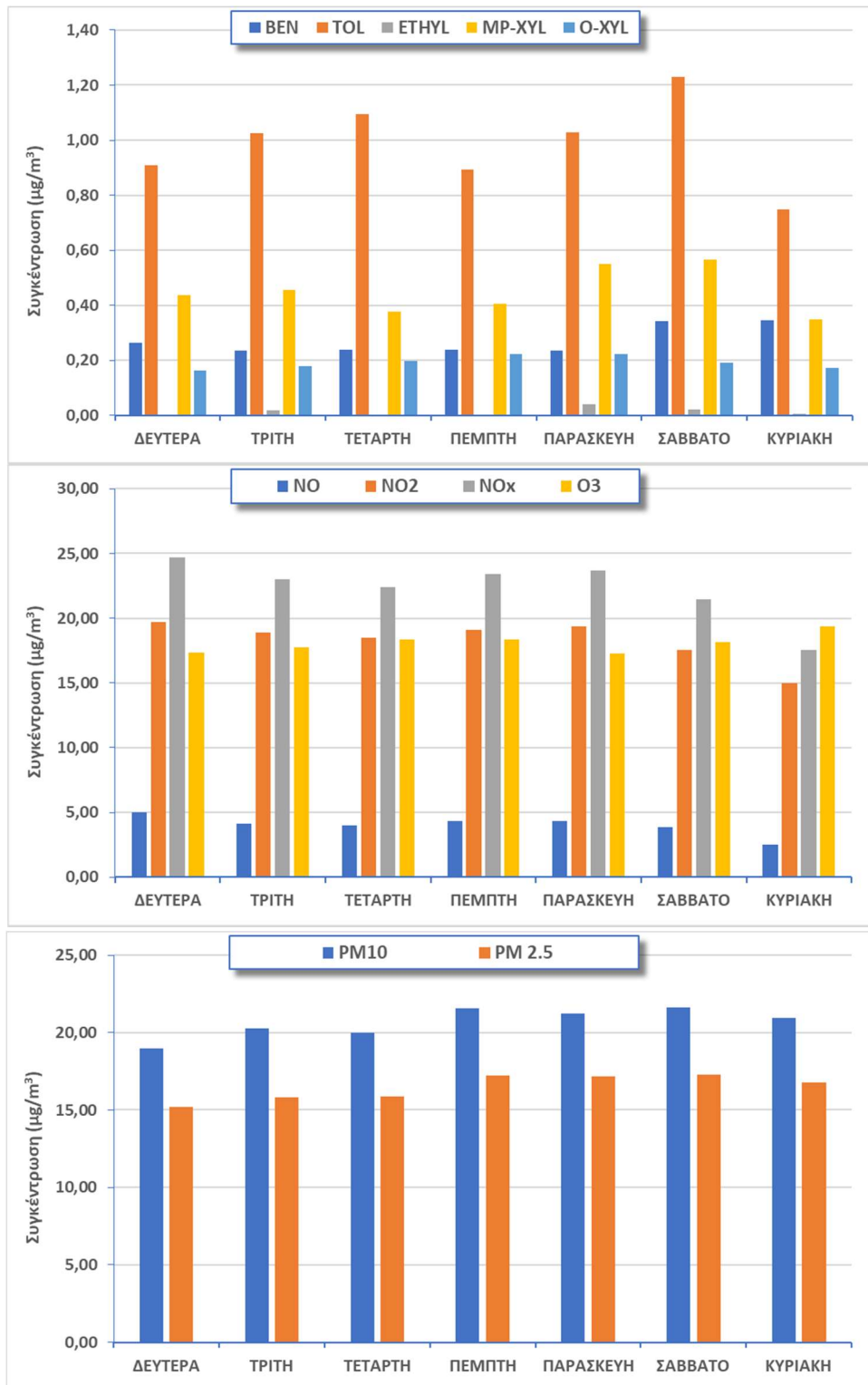
Σχήμα 2.1.2. Μέση εβδομαδιαία διακύμανση των συγκεντρώσεων BTEX, NOx, O 3 , PM 10 και PM 2.5 κατά το χρονικό διάστημα 02/06/2018 – 01/06/2019
