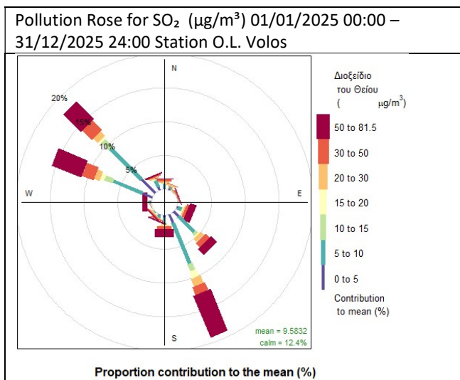
Σχήμα 2.1.5. Ροδογράμματα της % συμμετοχής των συγκεντρώσεων στον μέσο όρο των αέριων ρύπων (1h Average)
