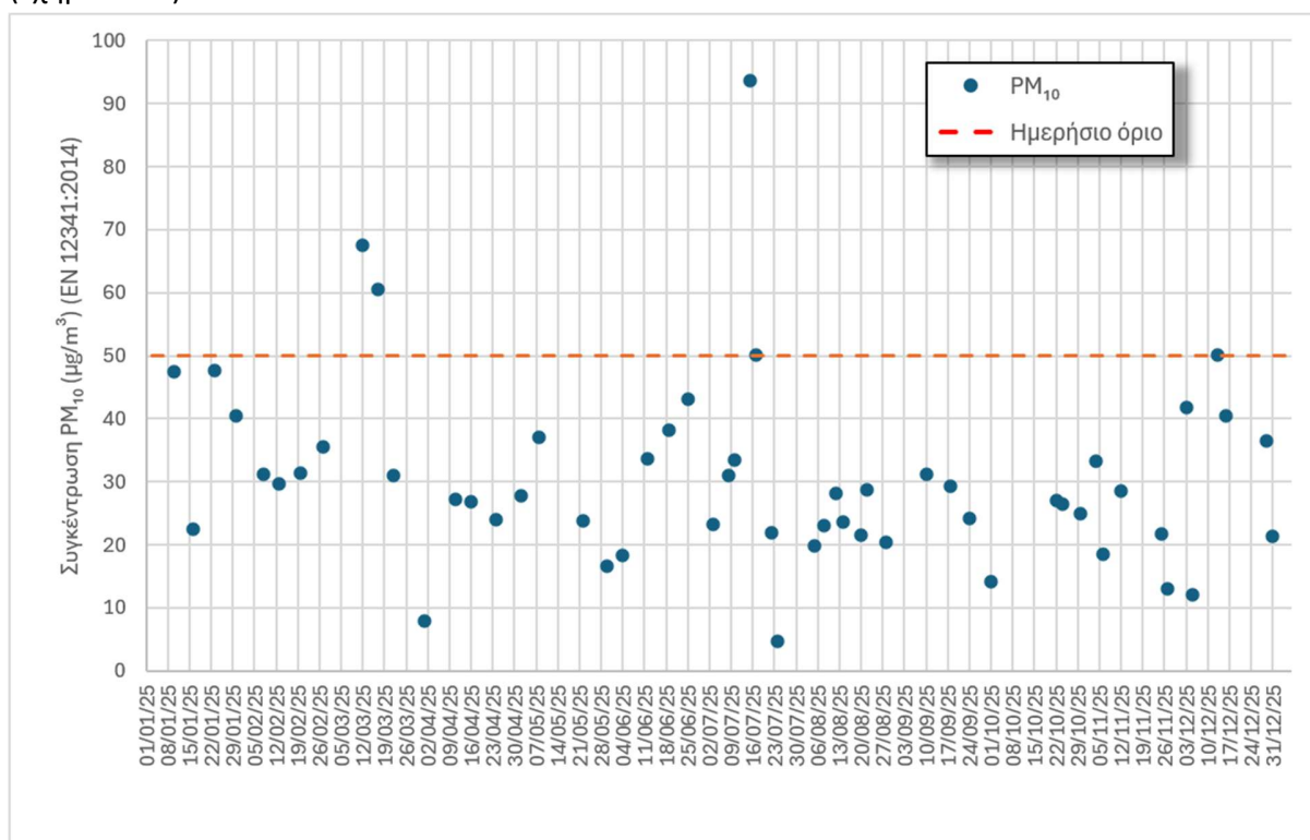
Σχήμα 2.2.1. Ημερήσιες σταθμικές συγκεντρώσεις PM 10 κατά το έτος 2025
