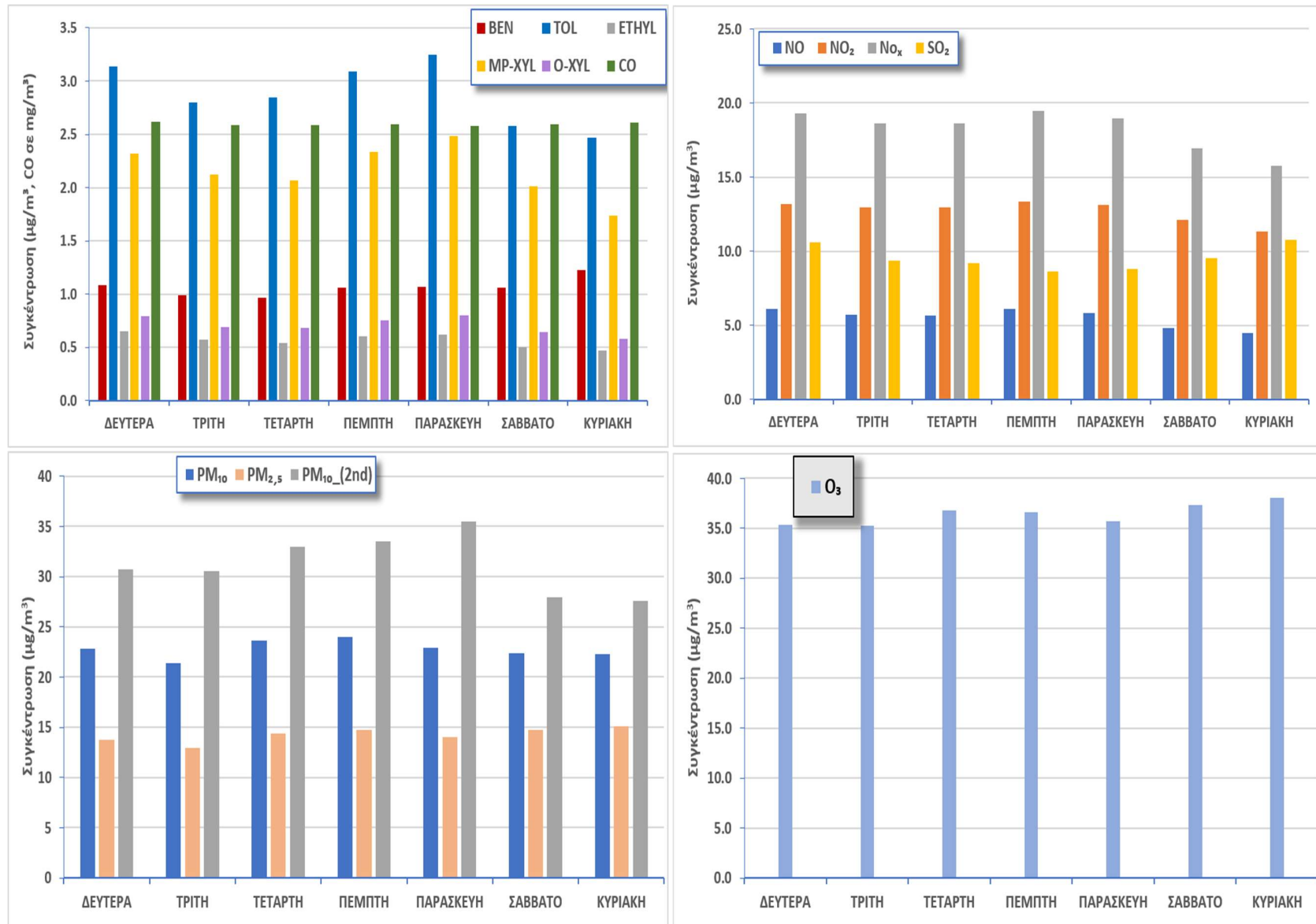
Σχήμα 2.1.2. Μέση εβδομαδιαία διακύμανση των συγκεντρώσεων BTEX, CO, NO x , SO 2 , O 3 , PM 10 και PM 2,5 κατά τη διάρκεια του έτους 2025
