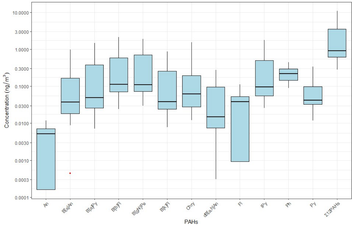
Σχήμα 2.2.2. Διάγραμμα box-and-whisker των συγκεντρώσεων PAHs ( ng/m^3 ) κατά το έτος 2025
