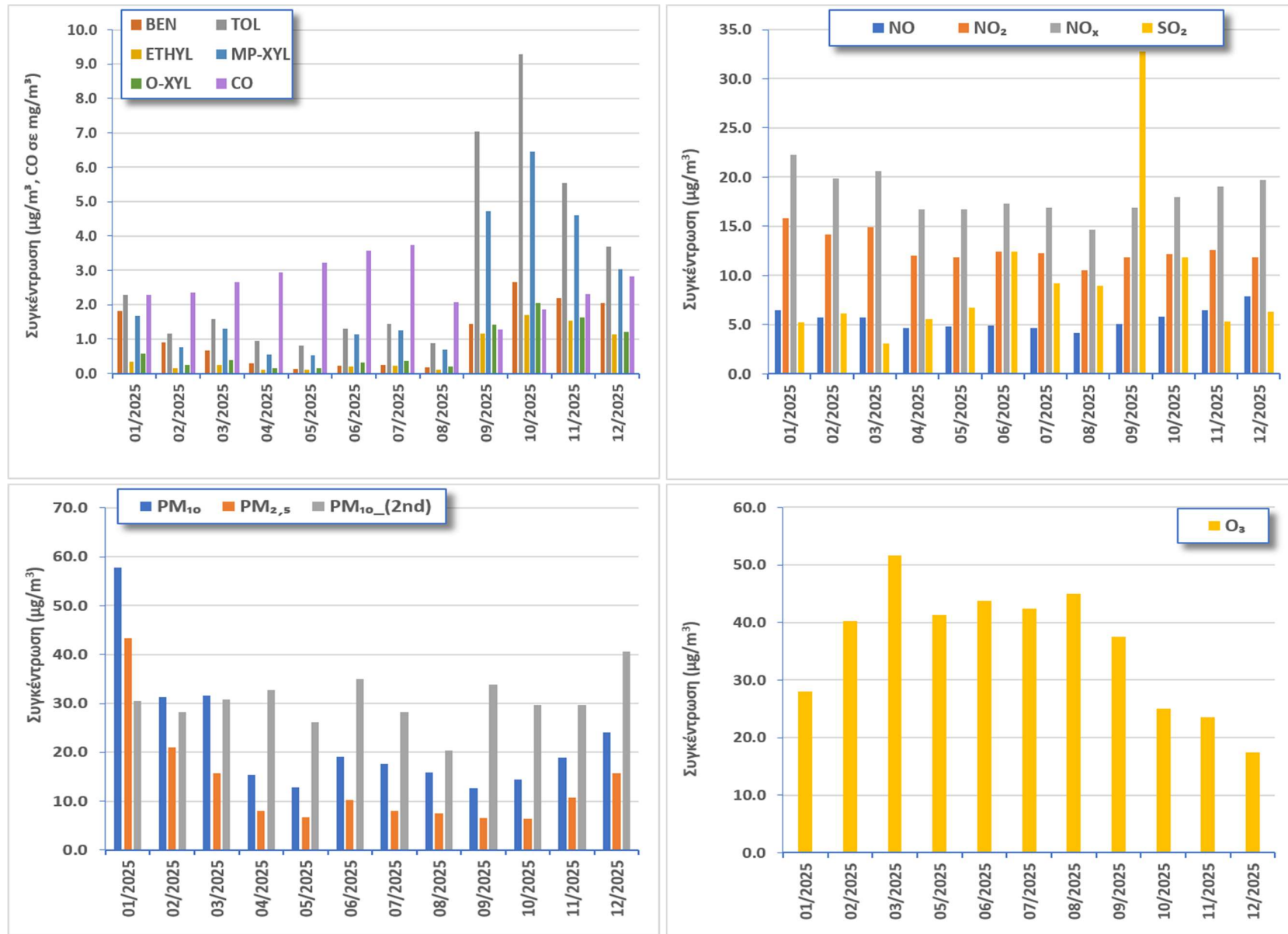
Σχήμα 2.1.3. Μέση μηνιαία διακύμανση των συγκεντρώσεων BTEX, CO, NO x , O 3 , PM 10 και PM 2,5 κατά τη διάρκεια του έτους 2025
