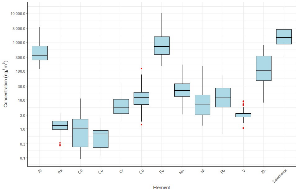
Σχήμα 2.2.3. Διάγραμμα box-and-whisker των συγκεντρώσεων μετάλλων / μεταλλοειδών ( ng/m^3 ) κατά το έτος 2025
