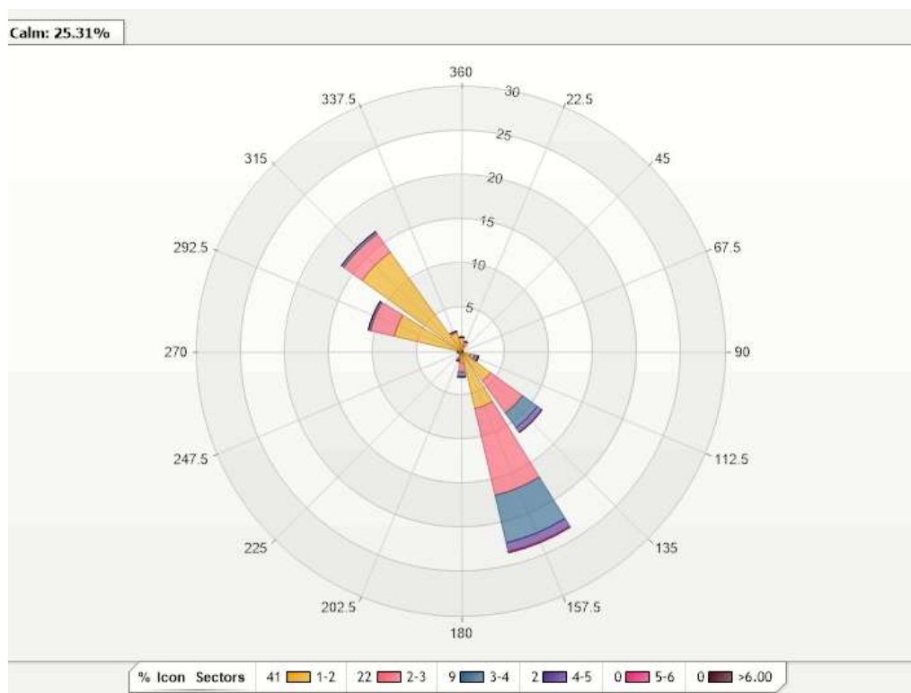
Σχήμα 2.1.4. Συχνότητα εμφάνισης και μέση ταχύτητα ανέμου ανά διεύθυνση προέλευσης κατά το έτος 2025
