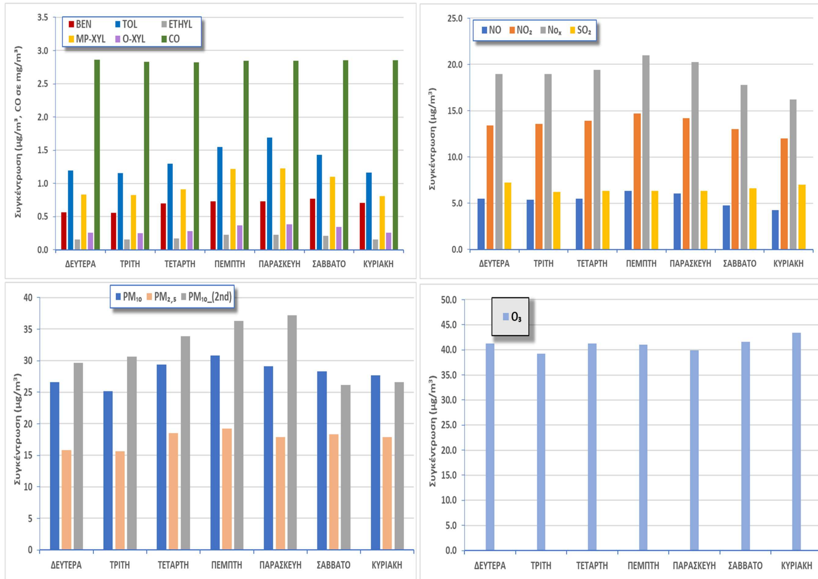
Σχήμα 2.1.2. Μέση εβδομαδιαία διακύμανση των συγκεντρώσεων BTEX, CO, NO x , SO 2 , O 3 , PM 10 και PM 2,5 κατά το χρονικό διάστημα 01.01.25 – 30.06.25
