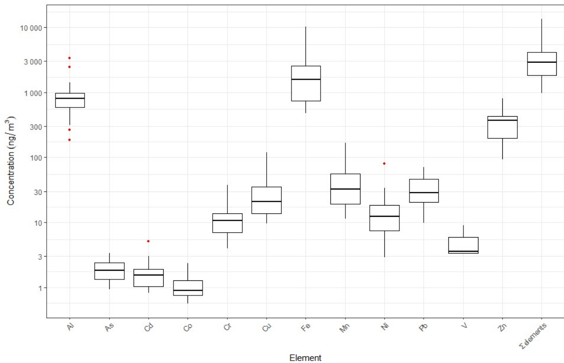
Σχήμα 2.2.3. Διάγραμμα box-and-whisker των συγκεντρώσεων μετάλλων / μεταλλοειδών ( ng/m^3 ) κατά το χρονικό διάστημα 01.01.25-30.06.25
