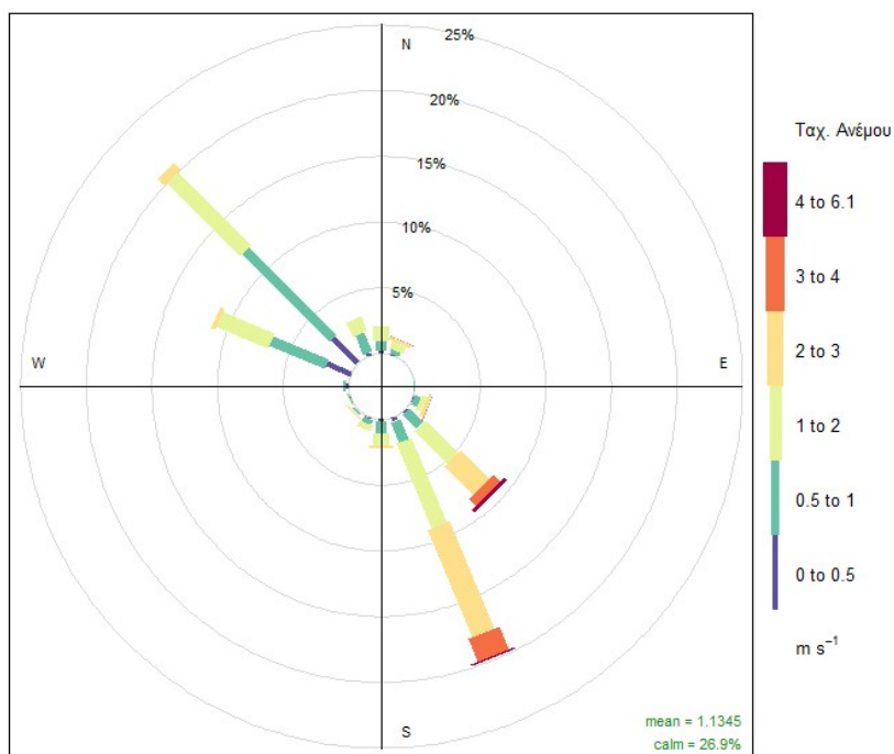
Σχήμα 2.1.4. Συχνότητα εμφάνισης και μέση ταχύτητα ανέμου ανά διεύθυνση προέλευσης κατά την περίοδο των μετρήσεων 01.01.25-30.06.25
