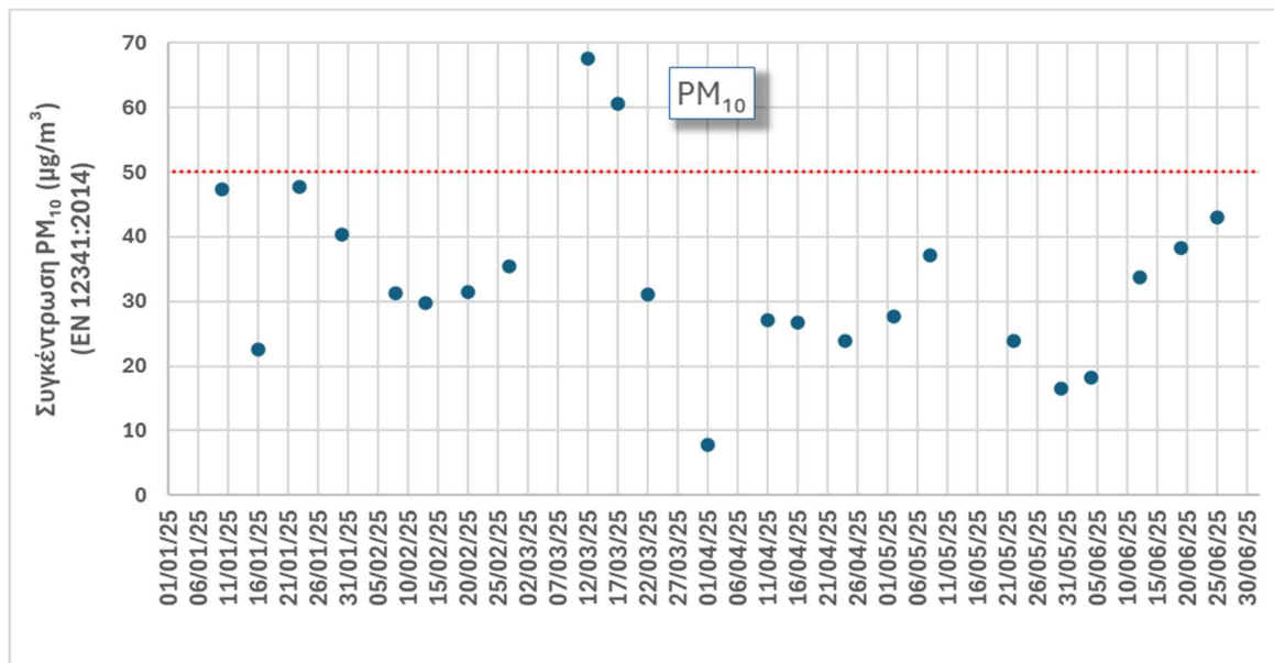
Σχήμα 2.2.1. Ημερήσιες σταθμικές συγκεντρώσεις PM 10 κατά το χρονικό διάστημα 01.01.25 – 30.06.25
