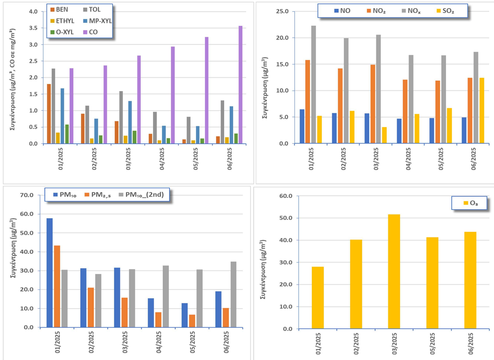
Σχήμα 2.1.3. Μέση μηνιαία διακύμανση των συγκεντρώσεων BTEX, CO, NO x , O 3 , PM 10 και PM 2,5 κατά το χρονικό διάστημα 01.01.25-30.06.25
