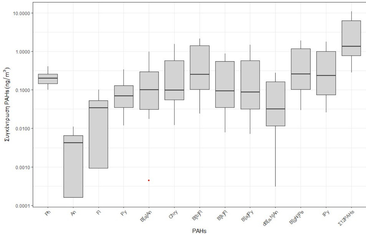
Σχήμα 2.2.2. Διάγραμμα box-and-whisker των συγκεντρώσεων PAHs ( ng/m^3 ) κατά το χρονικό διάστημα 01.01.25-30.06.25
