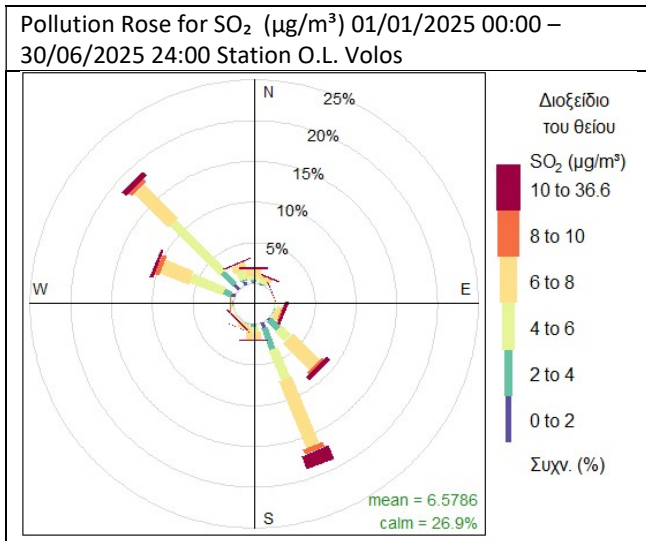
Σχήμα 2.1.5. Ροδογράμματα των συγκεντρώσεων των αέριων ρύπων (1h Average)
